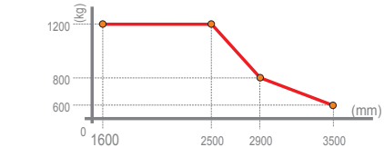
ALTURA DE ELEVAÇÃO x CAPACIDADE DE CARGA
